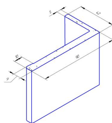
Рис. 9 Телескопический наличник L42
