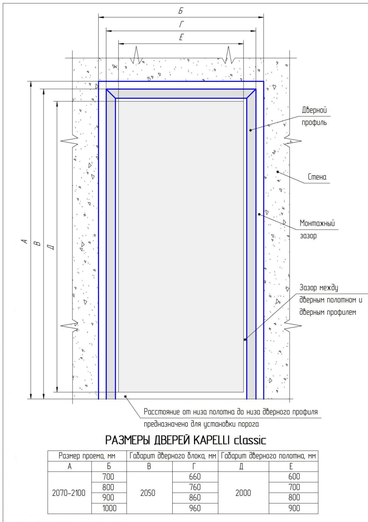
Рис. 26 Размеры стандартных дверных блоков.
